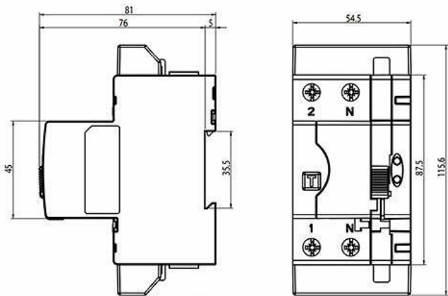
Figura 8: Dimensiones REC 4.
